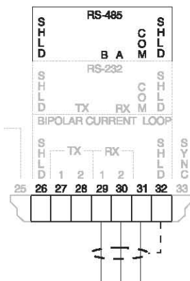
RS-485
